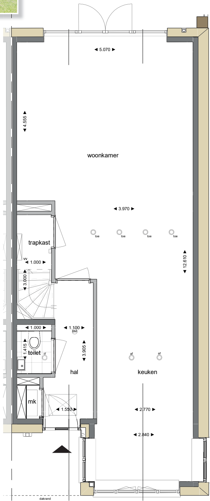
BEGANE GROND
