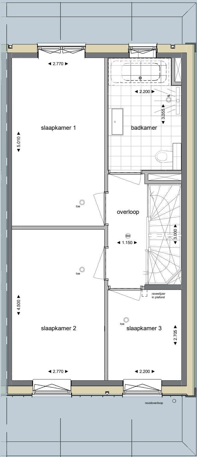
EERSTE VERDIEPING
