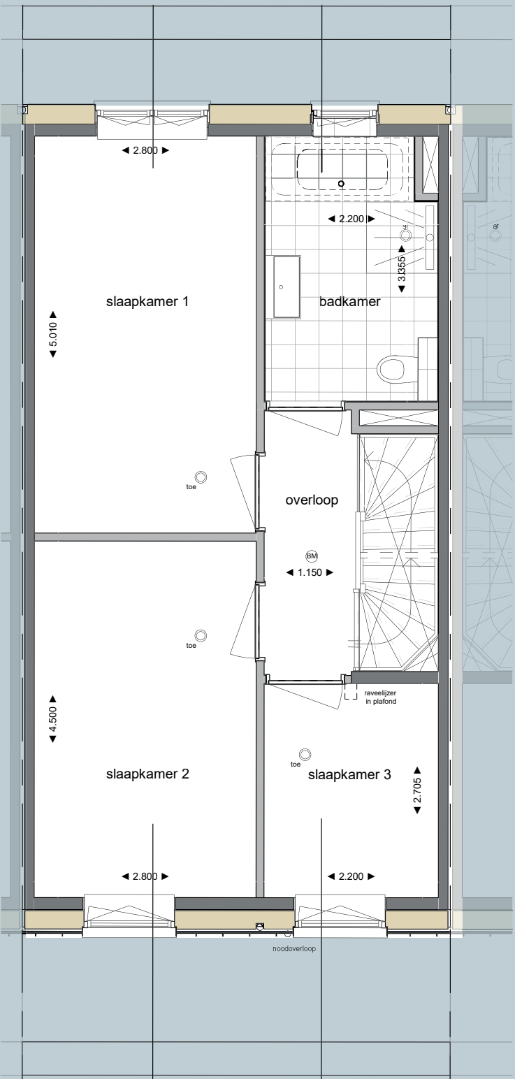
EERSTE VERDIEPING
