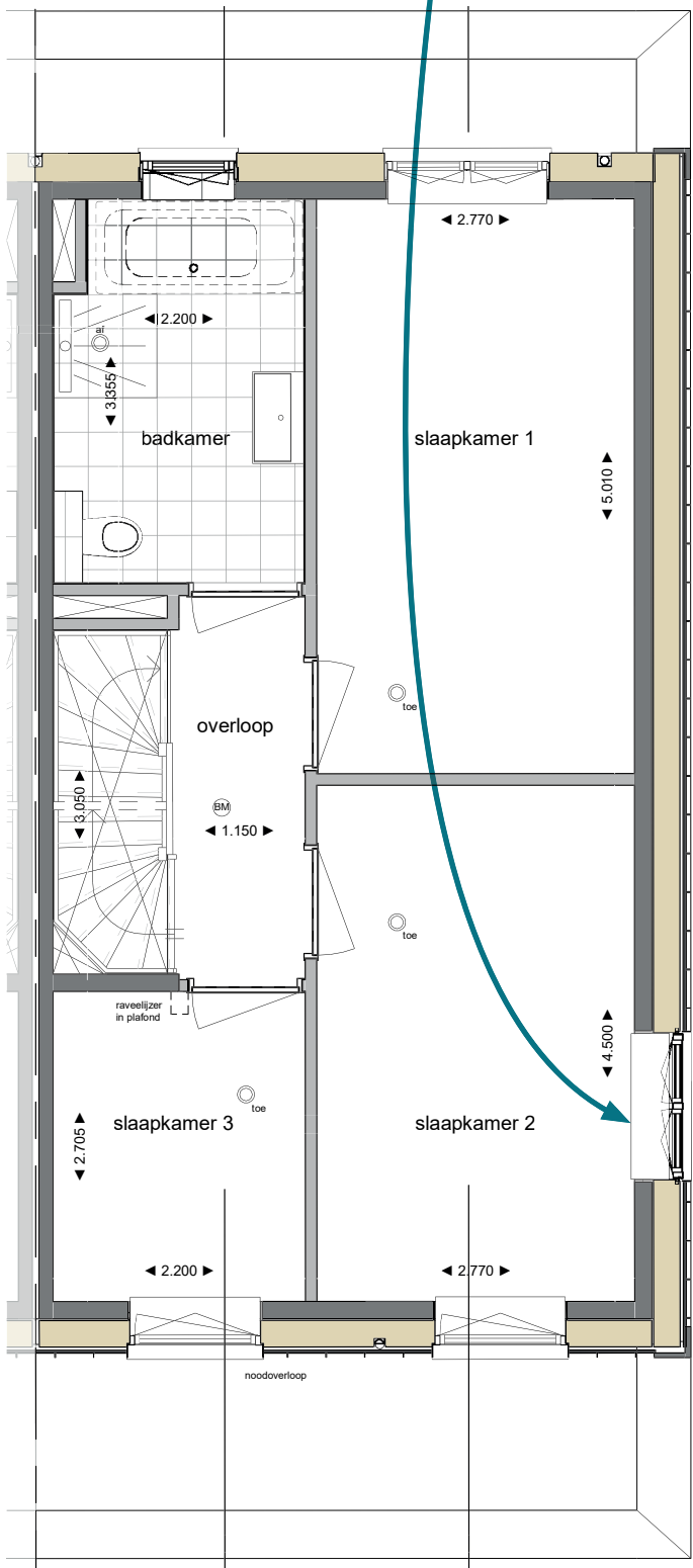
EERSTE VERDIEPING
