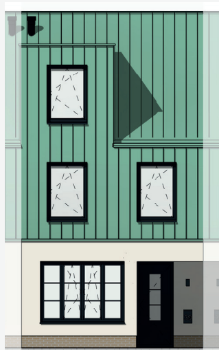
VOORAANZICHT
