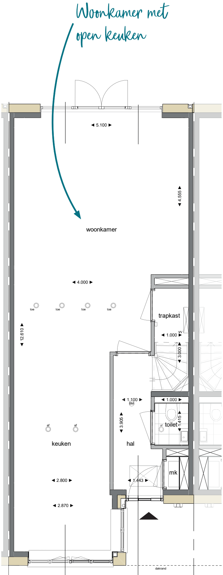
BEGANE GROND
