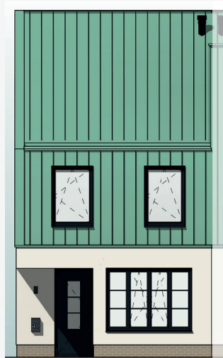
VOORAANZICHT
