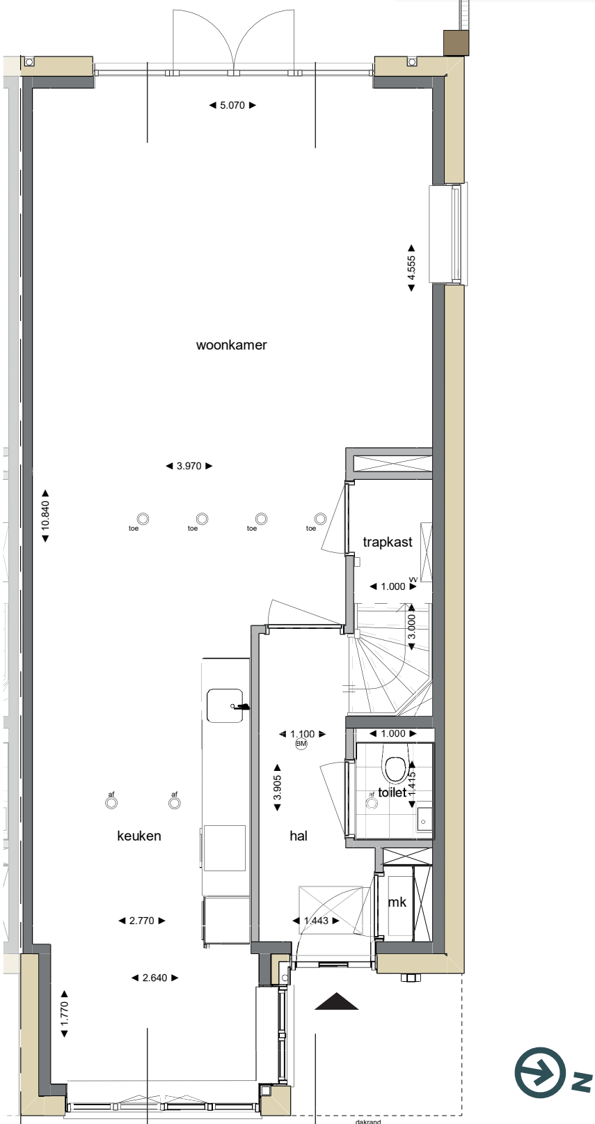
BEGANE GROND
