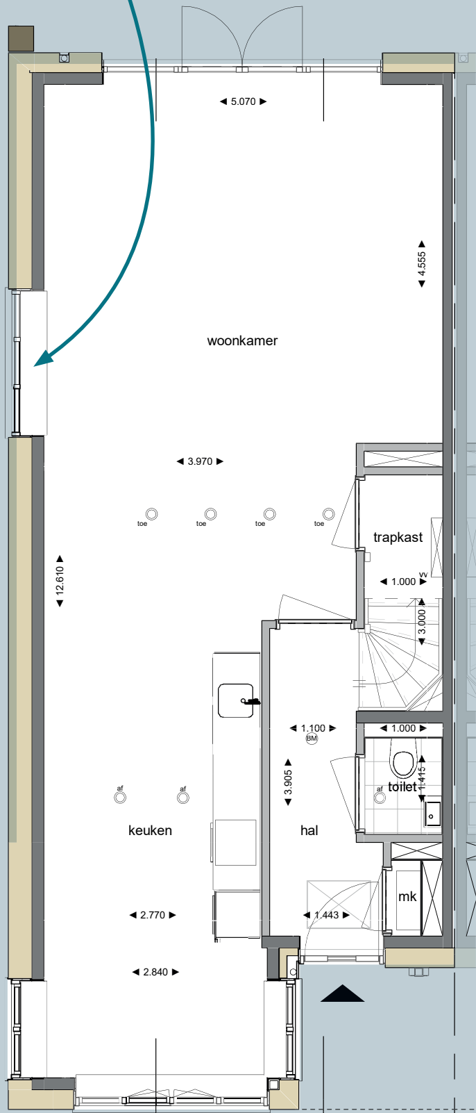
BEGANE GROND
