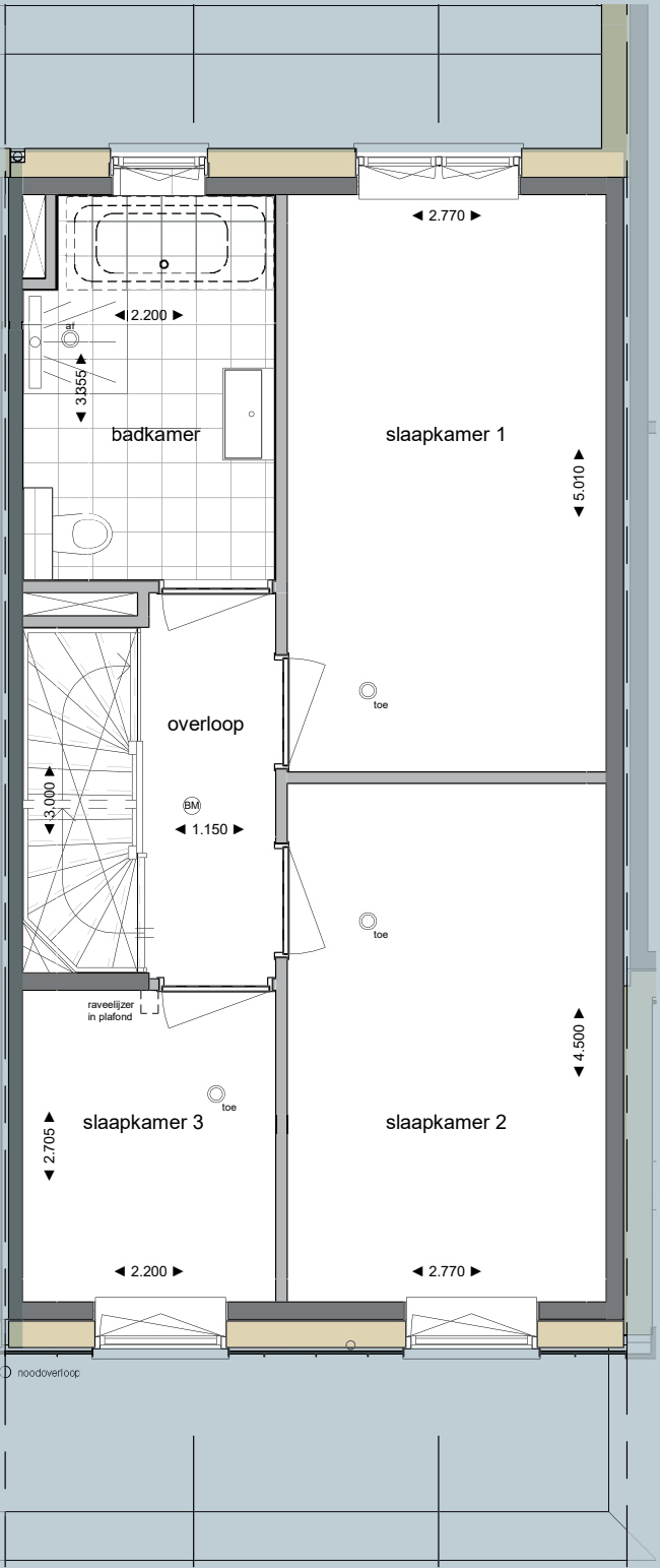
EERSTE VERDIEPING
