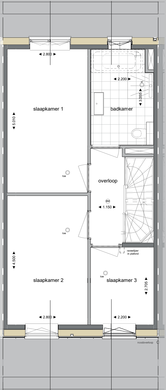
EERSTE VERDIEPING
